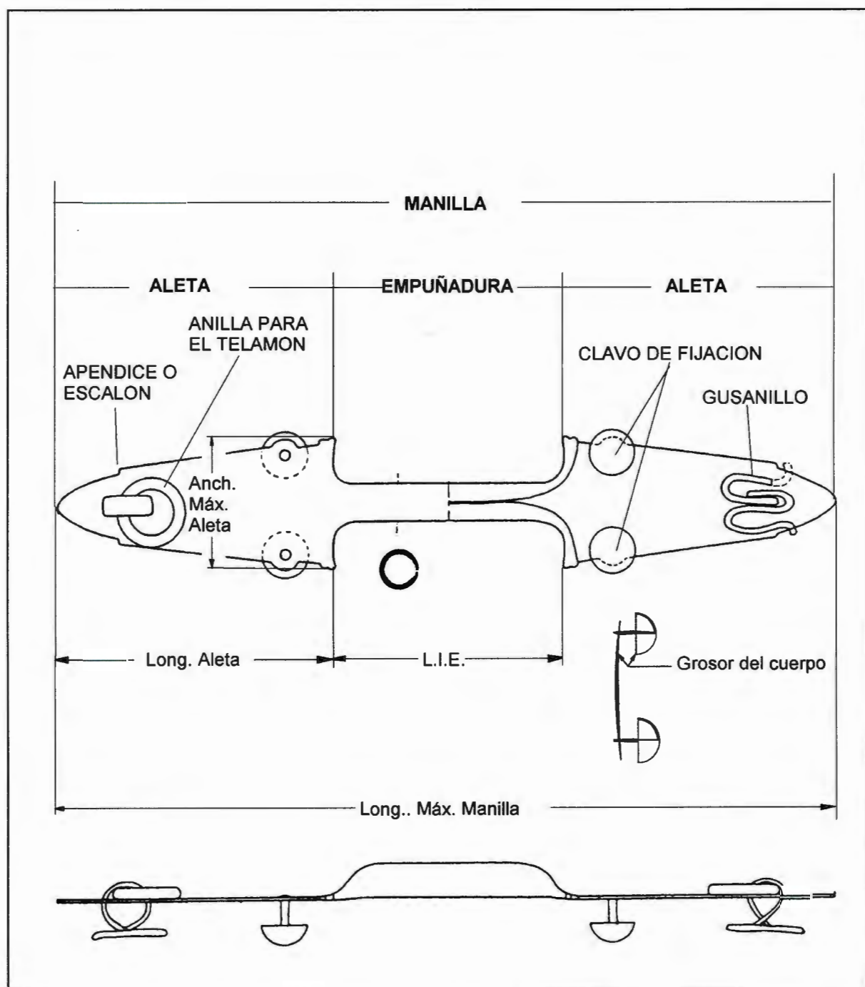
Figura: 287. Elementos y dimensiones básicas de una manilla de escudo de aletas ibérica.
