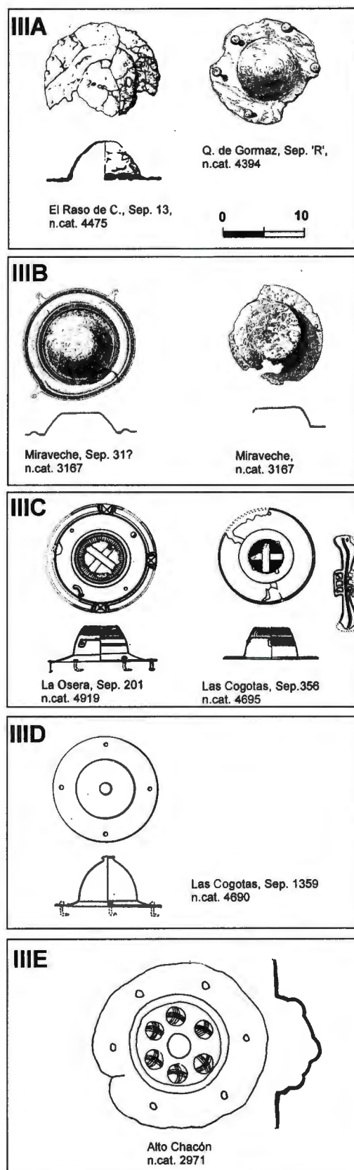
Figura: 298. Grupo III de umbos de escudo.
