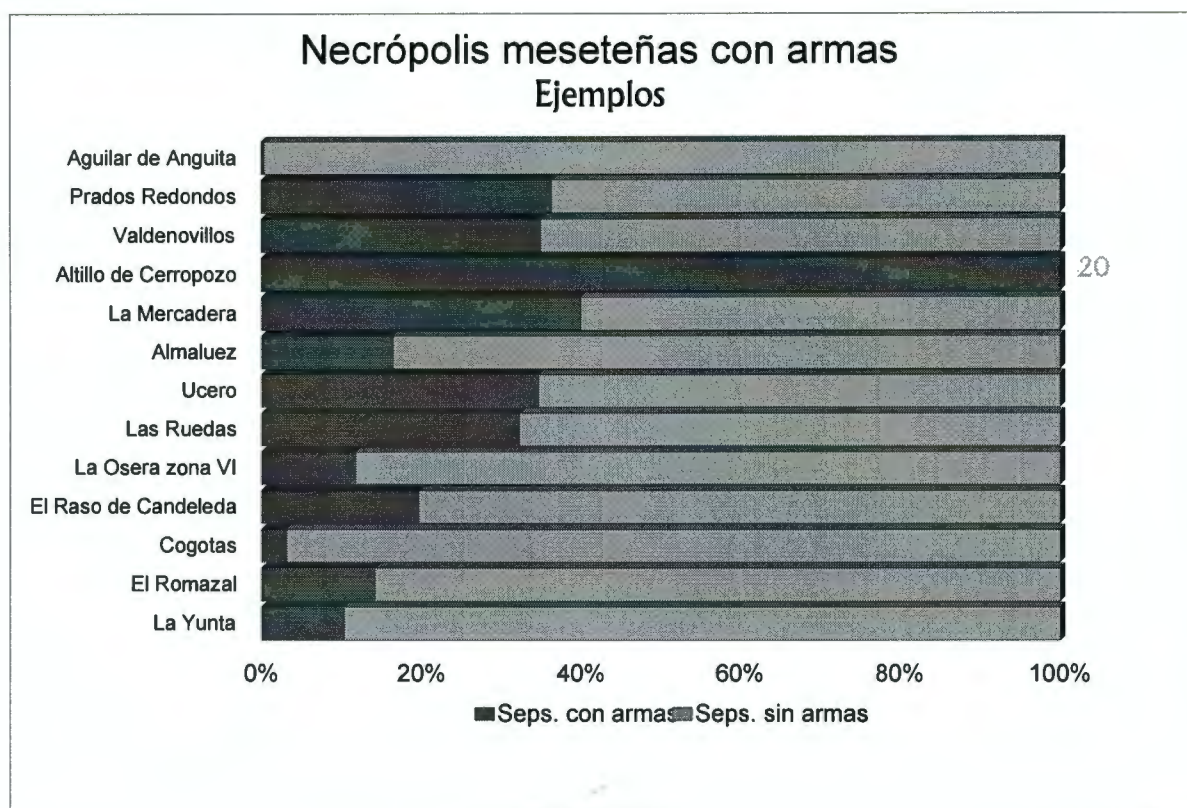
Figura: 347. Proporción de tumbas con armas en algunos yacimientos del interior peninsular.
