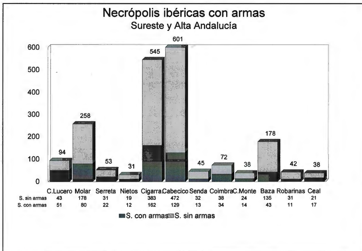
Figura: 346. Tumbas con armas en las principales necrópolis ibéricas del Sureste y Alta Andalucía. Valores absolutos.
