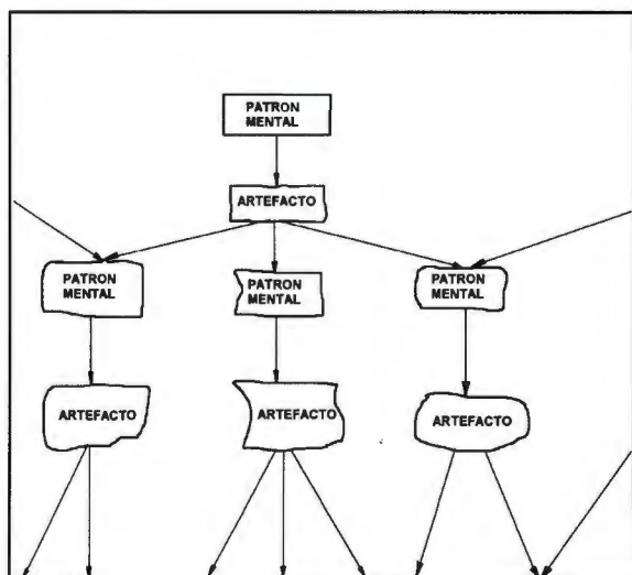
Figura: 336. 'Patrones mentales' en la creación de armas y la difusión de ideas entre los artesanos (según Bishop, 1987).
