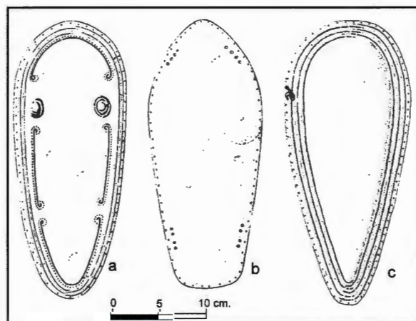
Figura: 334. Grebas metálicas de Aups, en el Sur de Francia (según Dehn).
