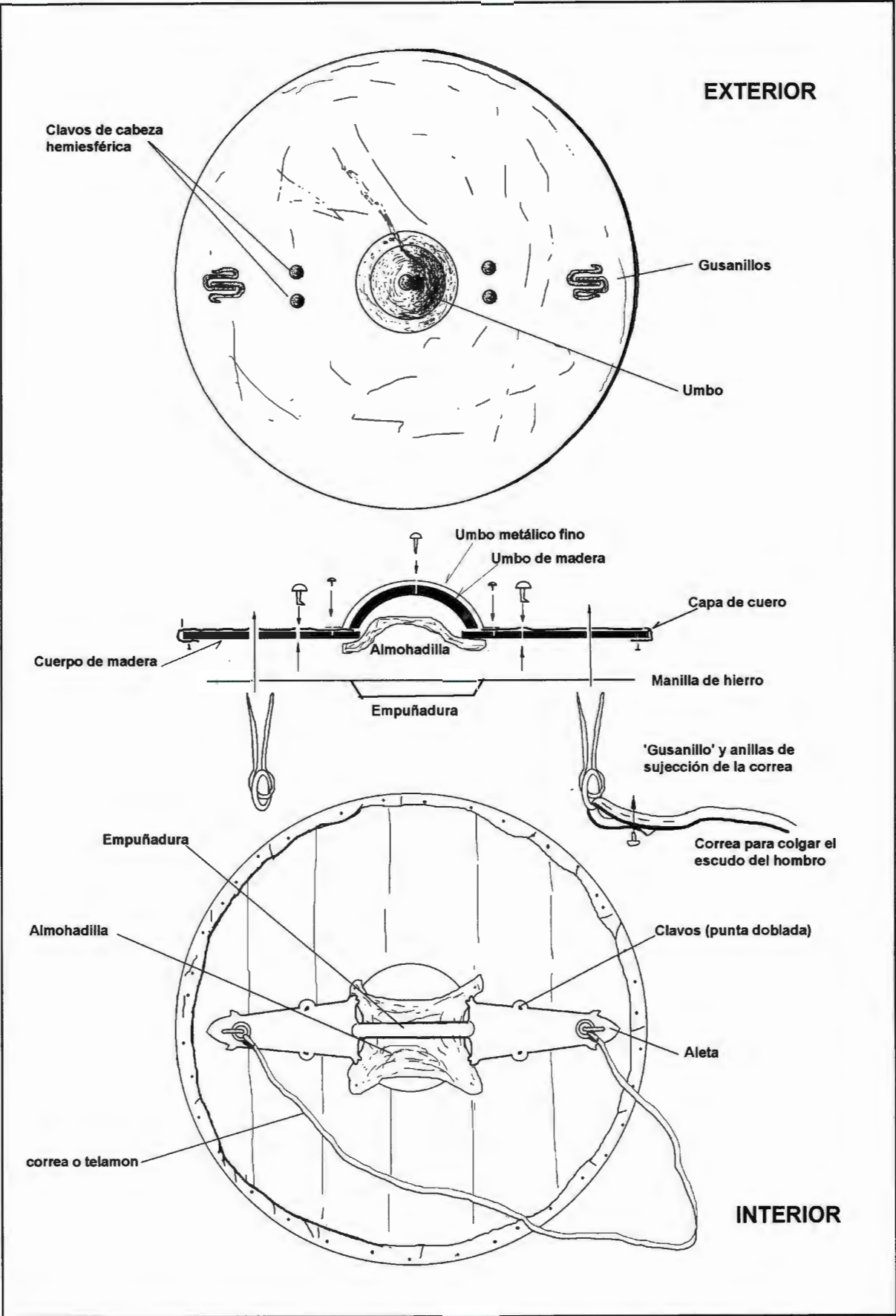
Figura: 286. Reconstrucción, elementos y denominación de la partes de un escudo circular ibérico con manilla de aletas.
