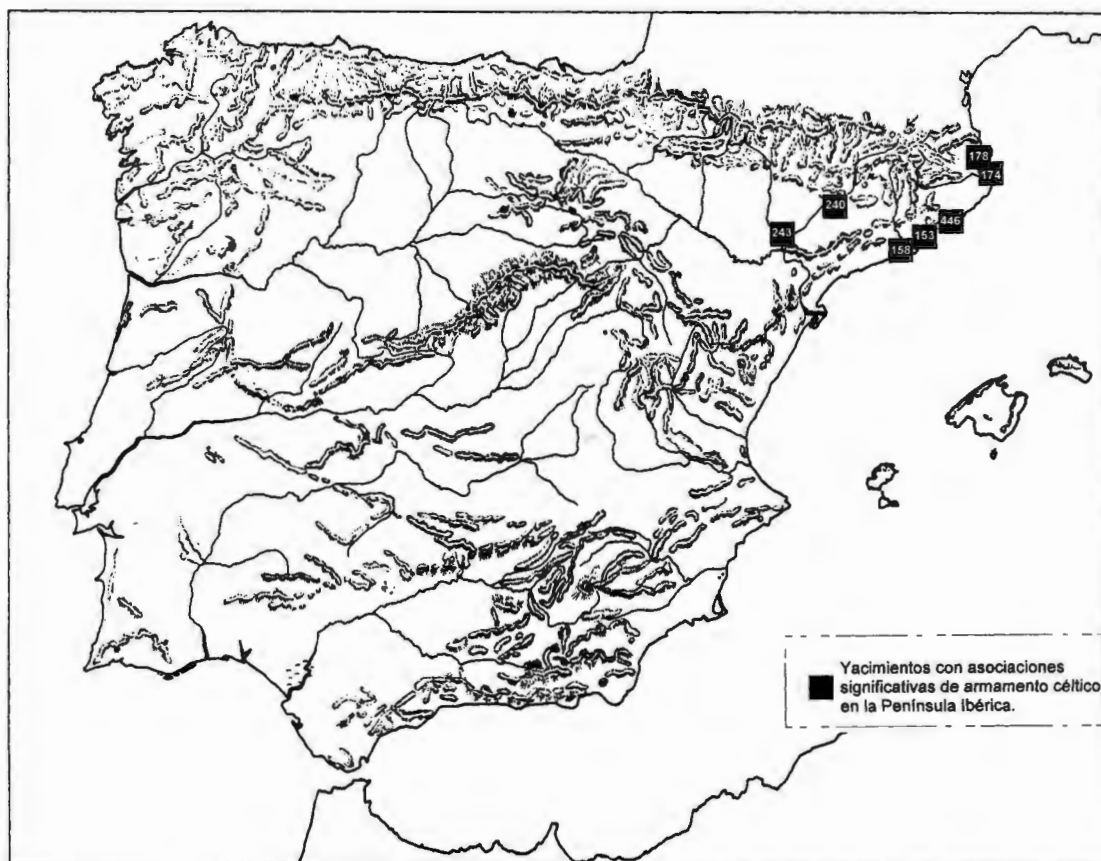
Figura: 343. Yacimientos con asociaciones significativas de armamento de tipo galo de La Tène (espadas de La Tène 'verdaderas' y umbos de escudo oval de tipo céltico, o espadas y cascos celtas y lanzas de tipo laténico).
