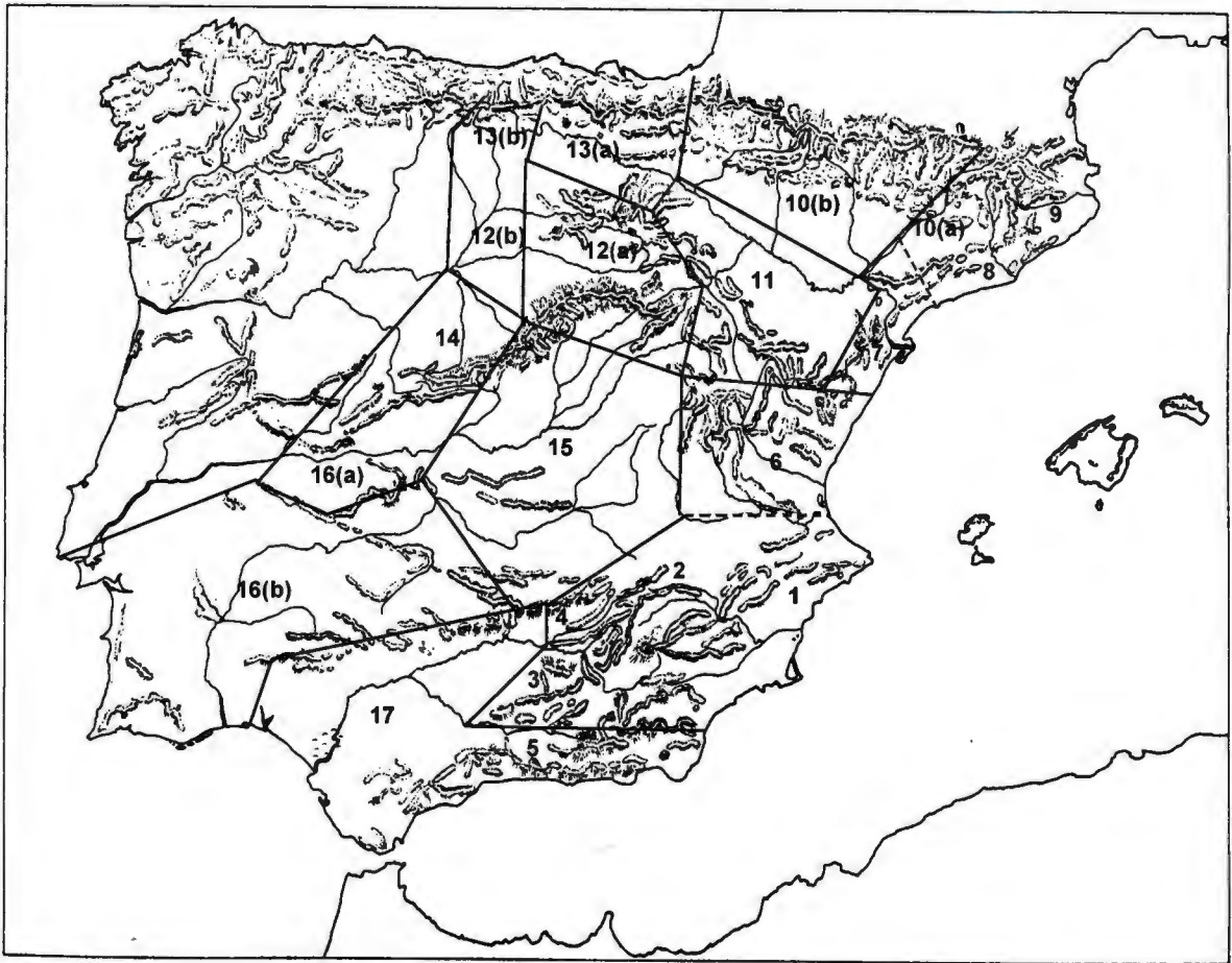
Figura: 342. Peculiaridades regionales del armamento prerromano. Zonas definidas y zonas con falta de información. Las fronteras son aproximadas.
