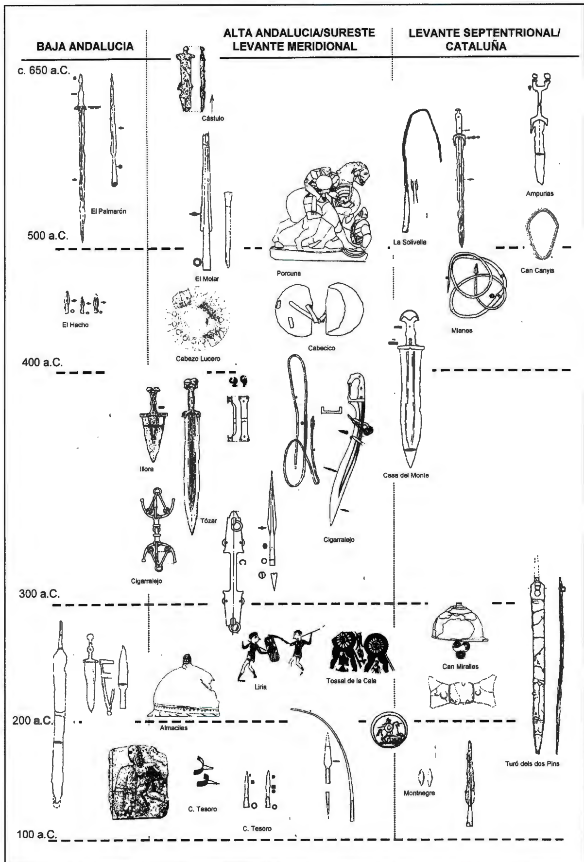
Figura: 337. Cuadro general simplificado de evolución de la panoplia ibérica por épocas y por regiones.
