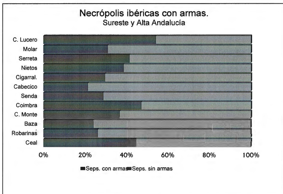
Figura: 345. Porcentajes de sepulturas con armas en algunas necrópolis del Sureste y Alta Andalucía.
