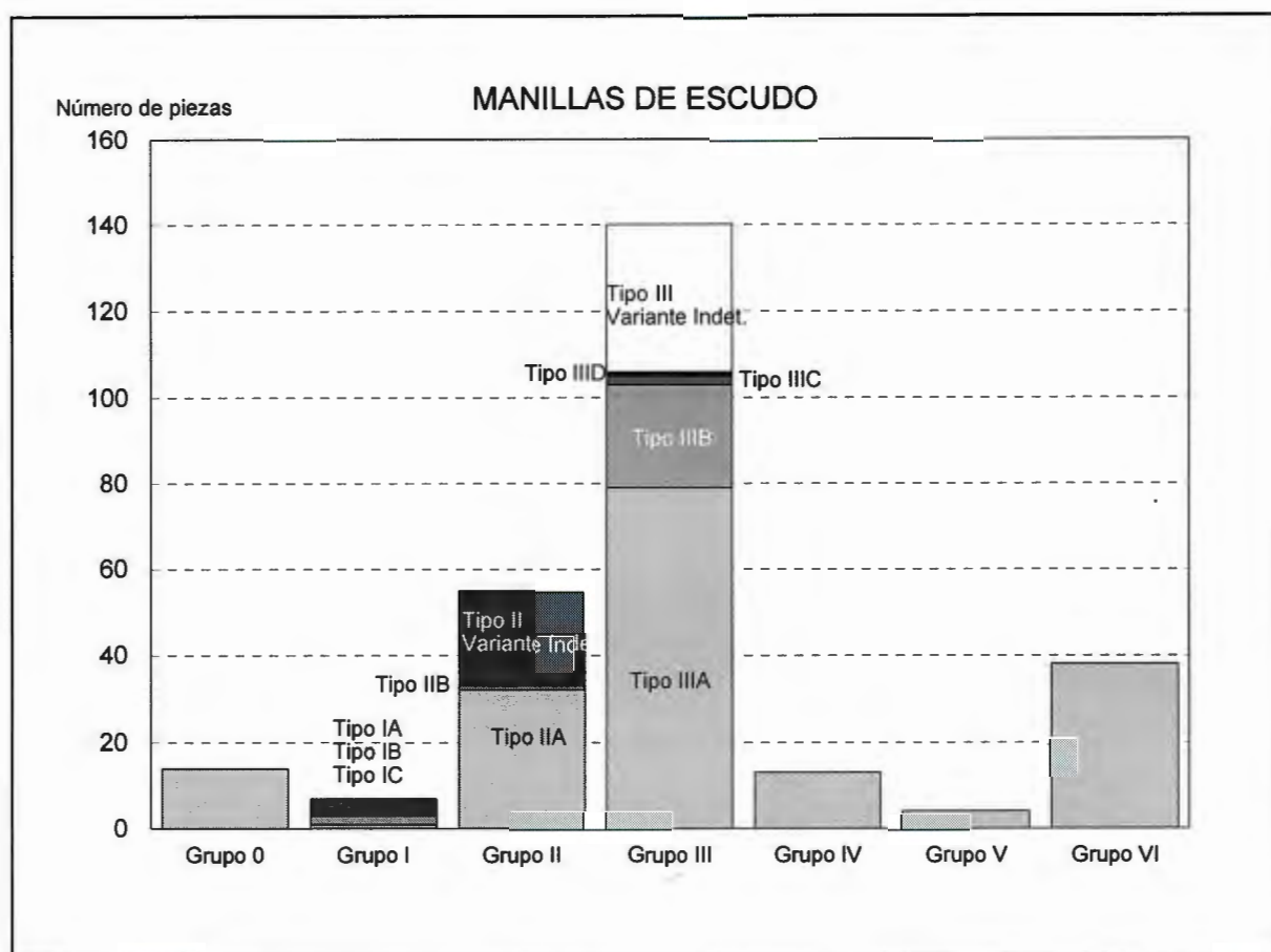
Figura: 292. Número de ejemplares de los distintos grupos de manilla de escudo.
