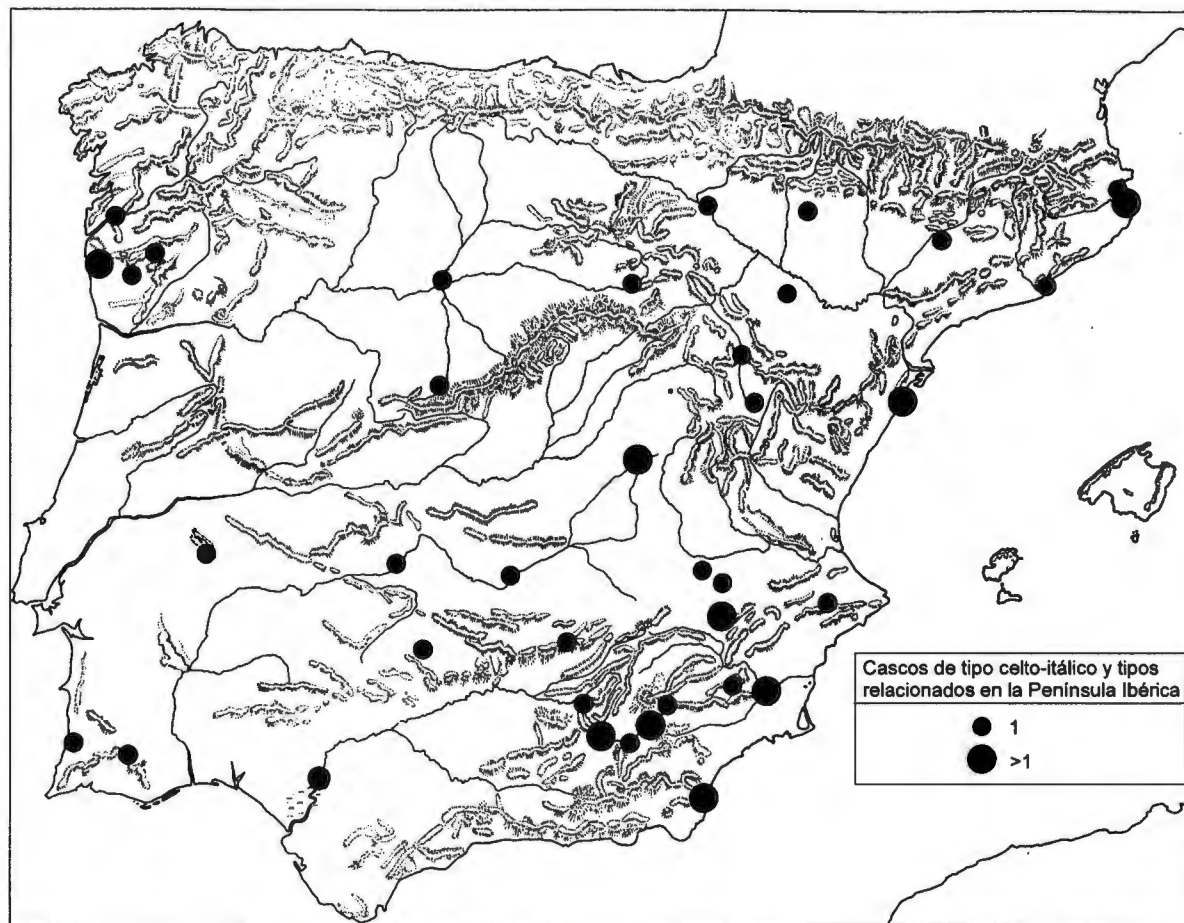
Figura: 319. Mapa de distribución 'mudo' de los cascos de tipo Montefortino y otros tipos relacionados. La distribución resulta incomprensible si no se tiene en cuenta contexto y cronología.
