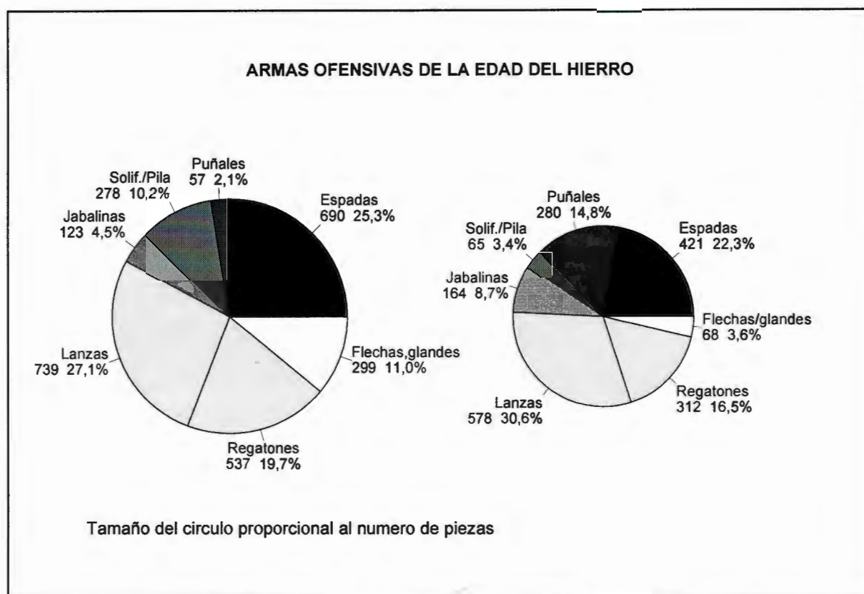
Figura: 354. Proporciones de los diversos tipos de armas ofensivas en el mundo ibérico (izquierda) y la Meseta (derecha).
