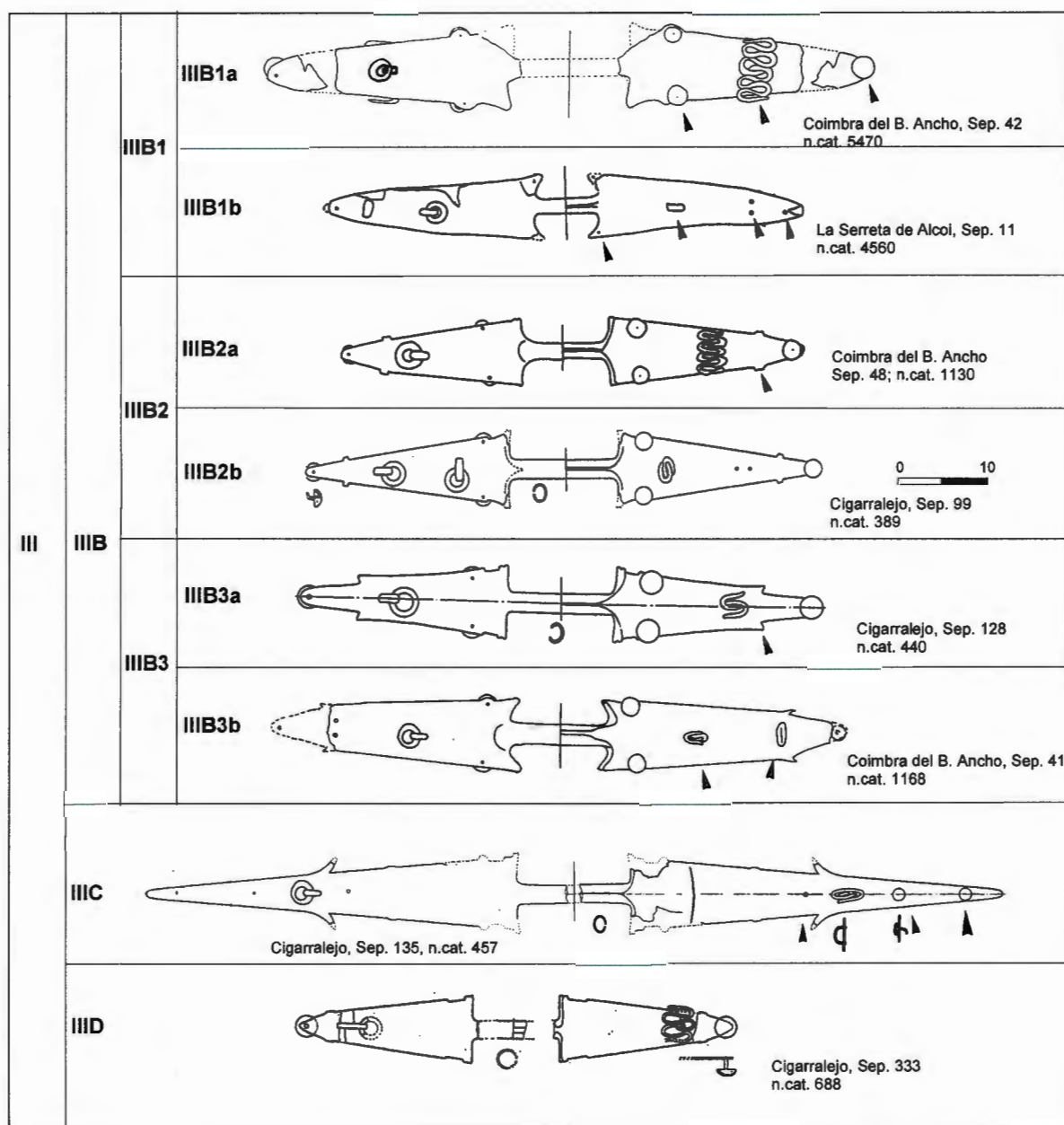
Figura: 290. Tipología de las manillas metálicas de escudo ibéricas.
