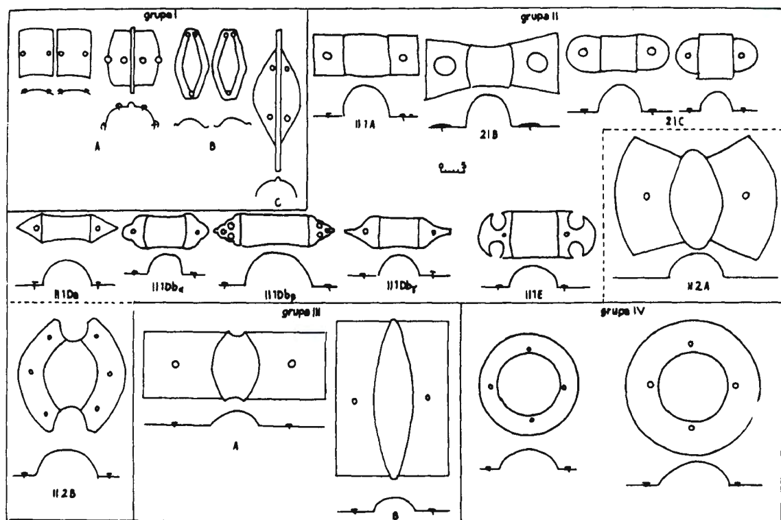
Figura: 311. Evolución de umbos de escudo oval en Europa central (según Domaradzki).
